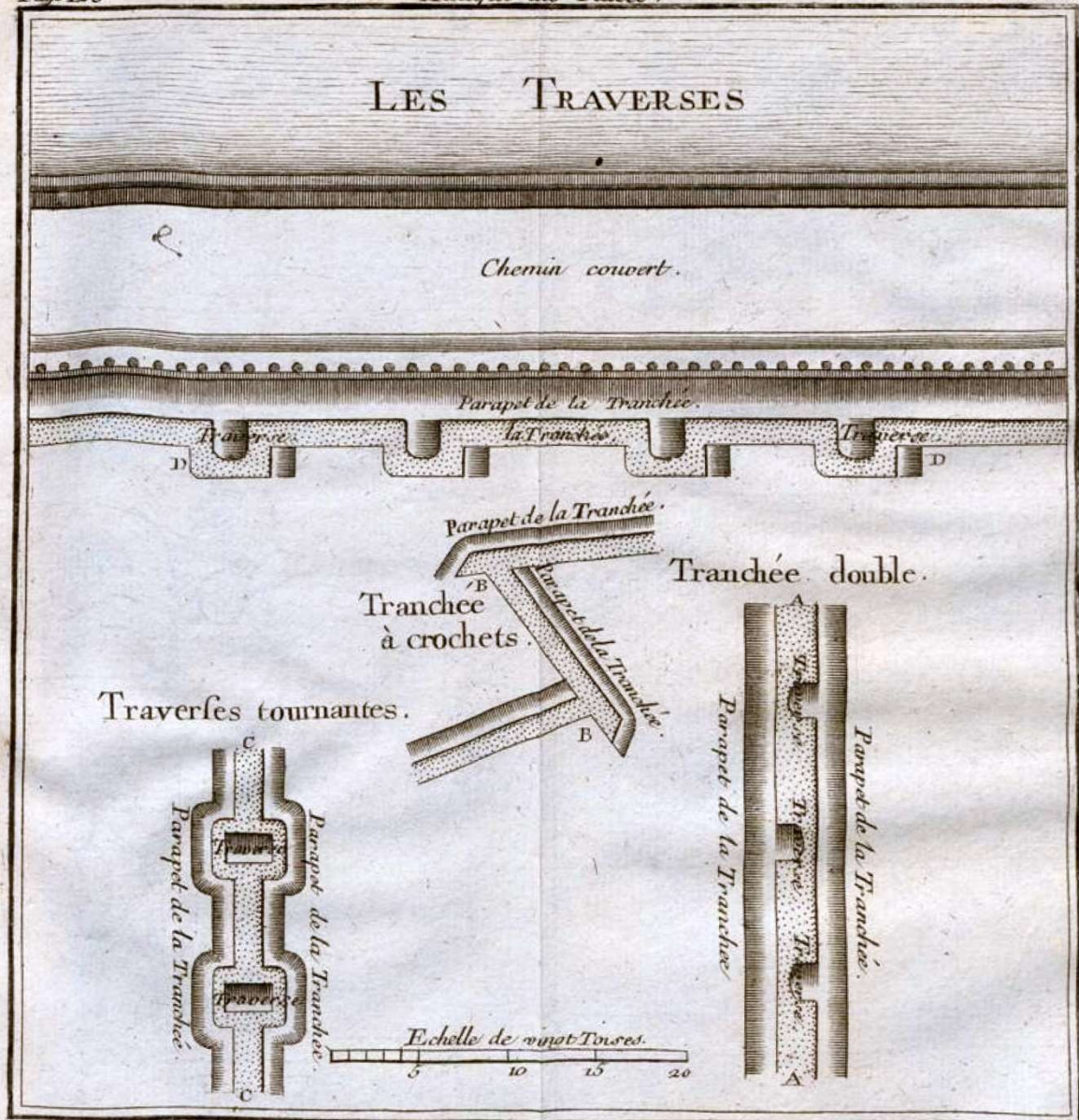
Abbildung 5: Die Sappen (Laufgräben) aus der Vogelschau, von oben nach unten: am gedeckten Weg der Festung, Zick-Zack der Approchen (Annäherungsgräben), Würfelsappen und doppelte Sappe
