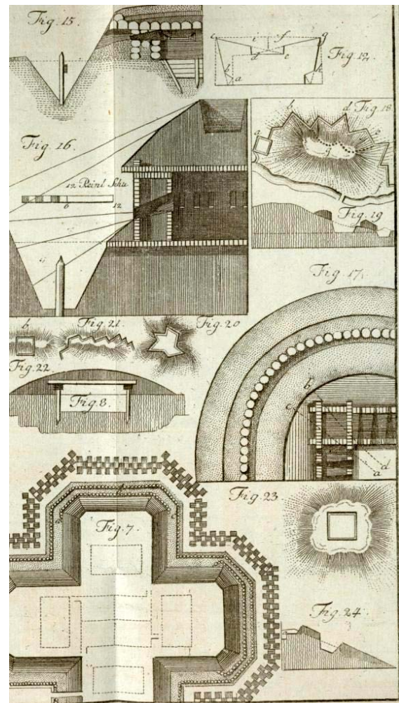
Abbildung 6: Blockhäuser im Tracé (Fig. 7 und 17) und Profil (Fig. 15 und 16). Die geläufigste Form ist das Kreuzblockhaus in Fig. 7. Fig. 20 zeigt eine polygonale Feldbefestigung (Scharnhorst, Verschanzungskunst, Pl. 8).
