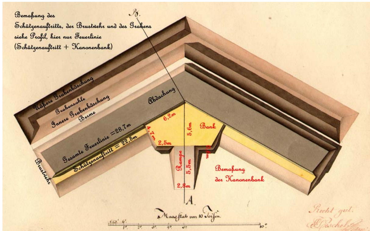
Abbildung 27: Tracé (Aufsicht) einer Flèche (Pfeilschanze; Redan) mit Bemaßungen in französischen Toisen (1 Klafter = 6 Fuß = ½ Ruthe), welche hier zum besseren Verständnis in metrische Angaben (schwarz für Feuerlinie, rot für Kanonenbank) umgerechnet sind. Von Oben nach unten: Schützenauftritt für die Infanterie, Brustwehr, Abdachung, innere Böschung, Berme, innere Grabenböschung, Grabensohle, äußere Grabenböschung. Im Ausspringenden Winkel liegt die leicht erhöhte Kanonenbank, damit das Geschütz über die Brustwehr feuern kann. Brustwehr, Schützenauftritt, Bank und Graben sind zur besseren Anschauung in verschiedenen Farben laviert. Maßstab der originalen Handzeichnung ca. 1:144 (Heinrich v. Witzleben, Eleve beim Adeligen Kadettencorps in Dresden, Prüfungsaufgaben ca. 1820).
