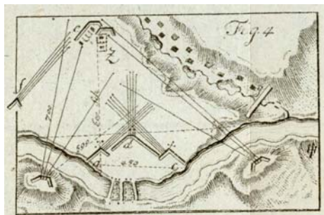
Abbildung 1: Einfachste Form eines Brückenkopfes als geschulterter Redan an einer einspringenden Flußschleife, so das Werk leicht von je einer Batterie des diesseitigen
