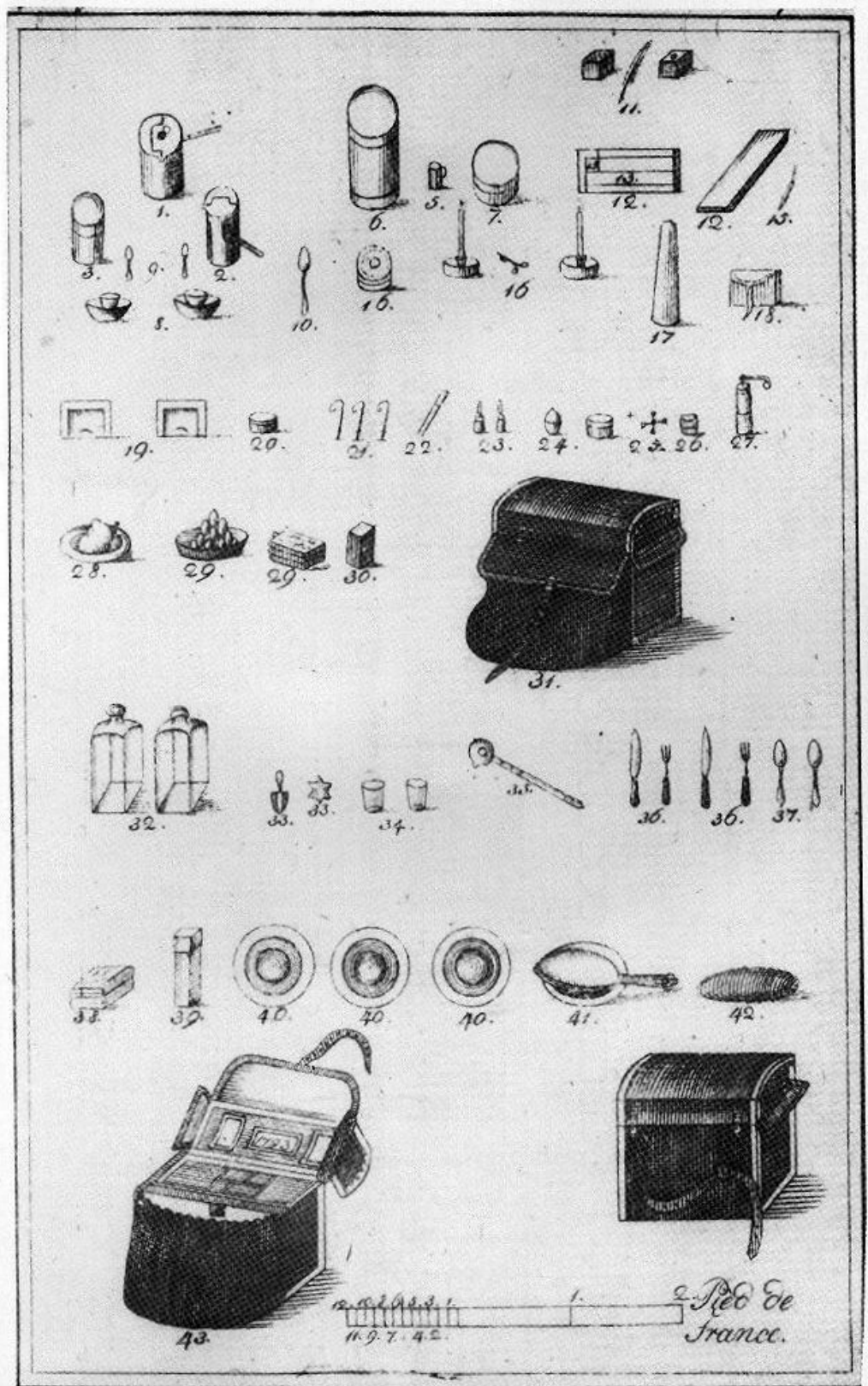
Tafel 95a: Feldkasten und Inhalt aus: Neueste Erfindung . . . (1794), Taf. 6
